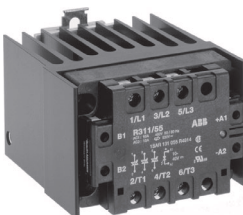
HDS 50/0,8
